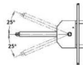
Deichsellenkung
