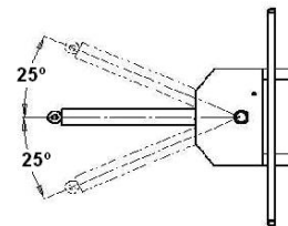
Deichsellenkung
